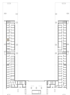
PLANTA ARRECADADAÇÃO PISO 5
