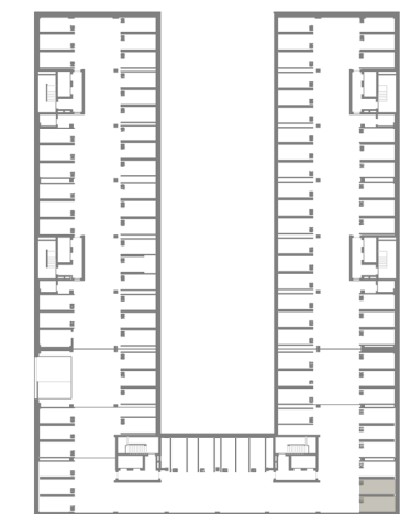
PLANTA ESTACIONAMENTO -1
