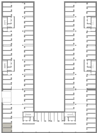
PLANTA ESTACIONAMENTO -1
