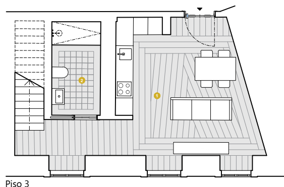
Piso 3
