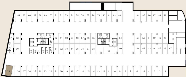
PLANTA PISO -2
