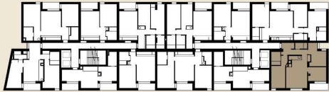
PLANTA PISO 2
