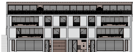
Fachada Rua
