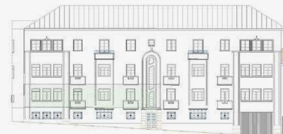
ALÇADO
