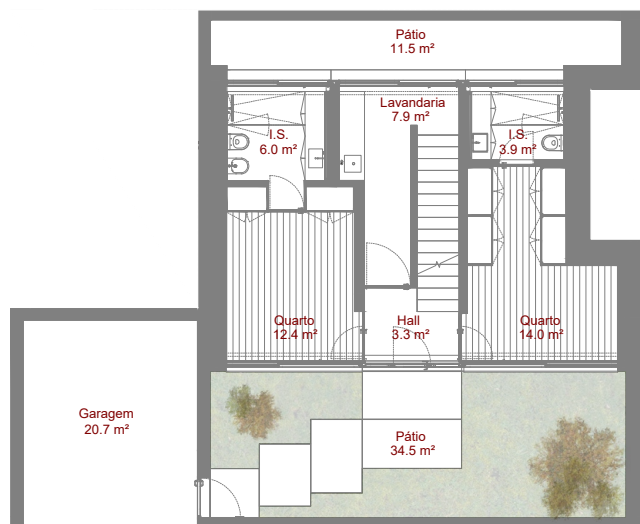
Planta Piso -1
