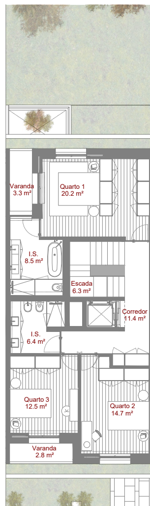
Planta Piso 1
