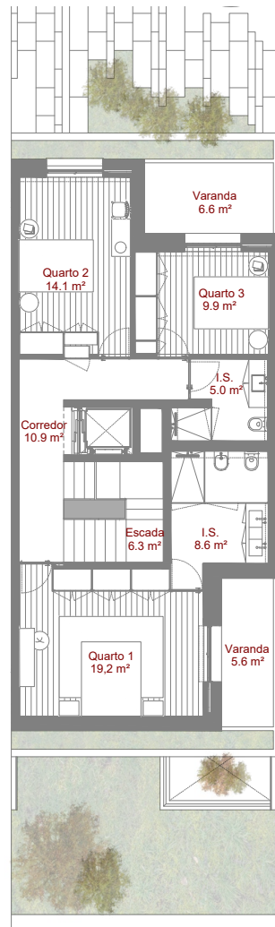
Planta Piso 1
