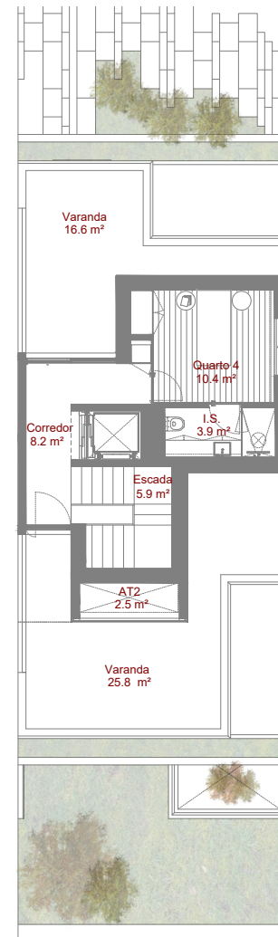
Planta Piso 2
