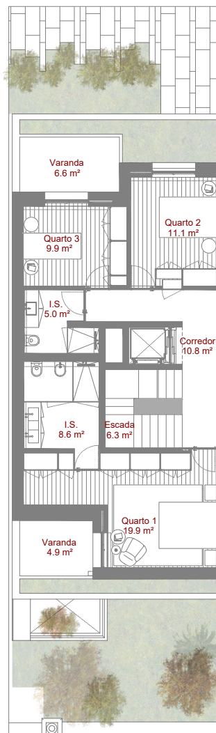
Planta Piso 1
