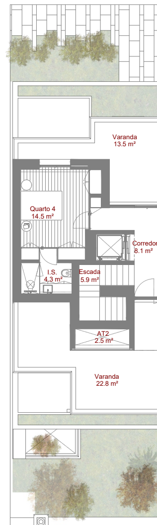
Planta Piso 2
