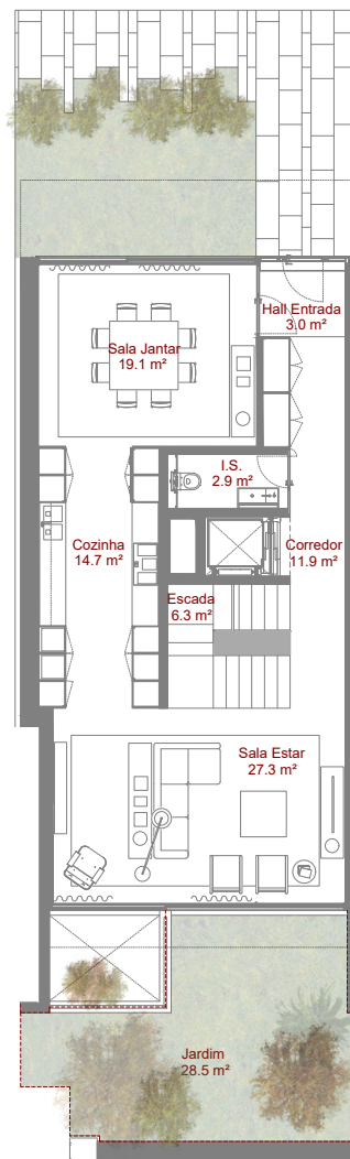
Planta Piso 0
