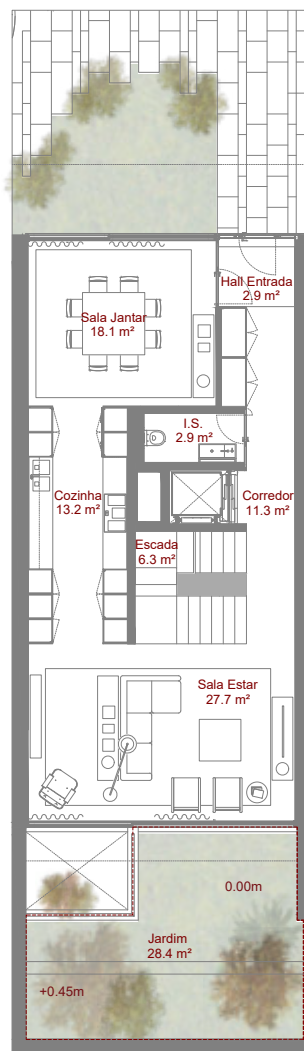
Planta Piso 0
