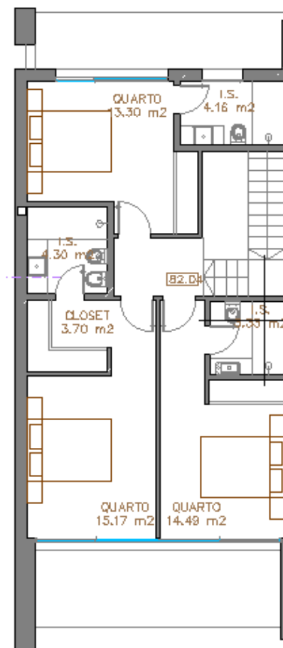
Planta - Piso 1
