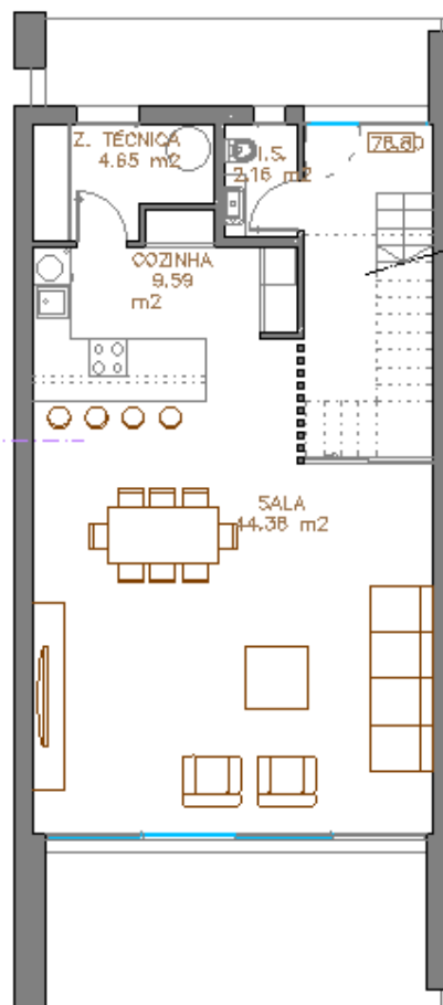
Planta - Piso 0
