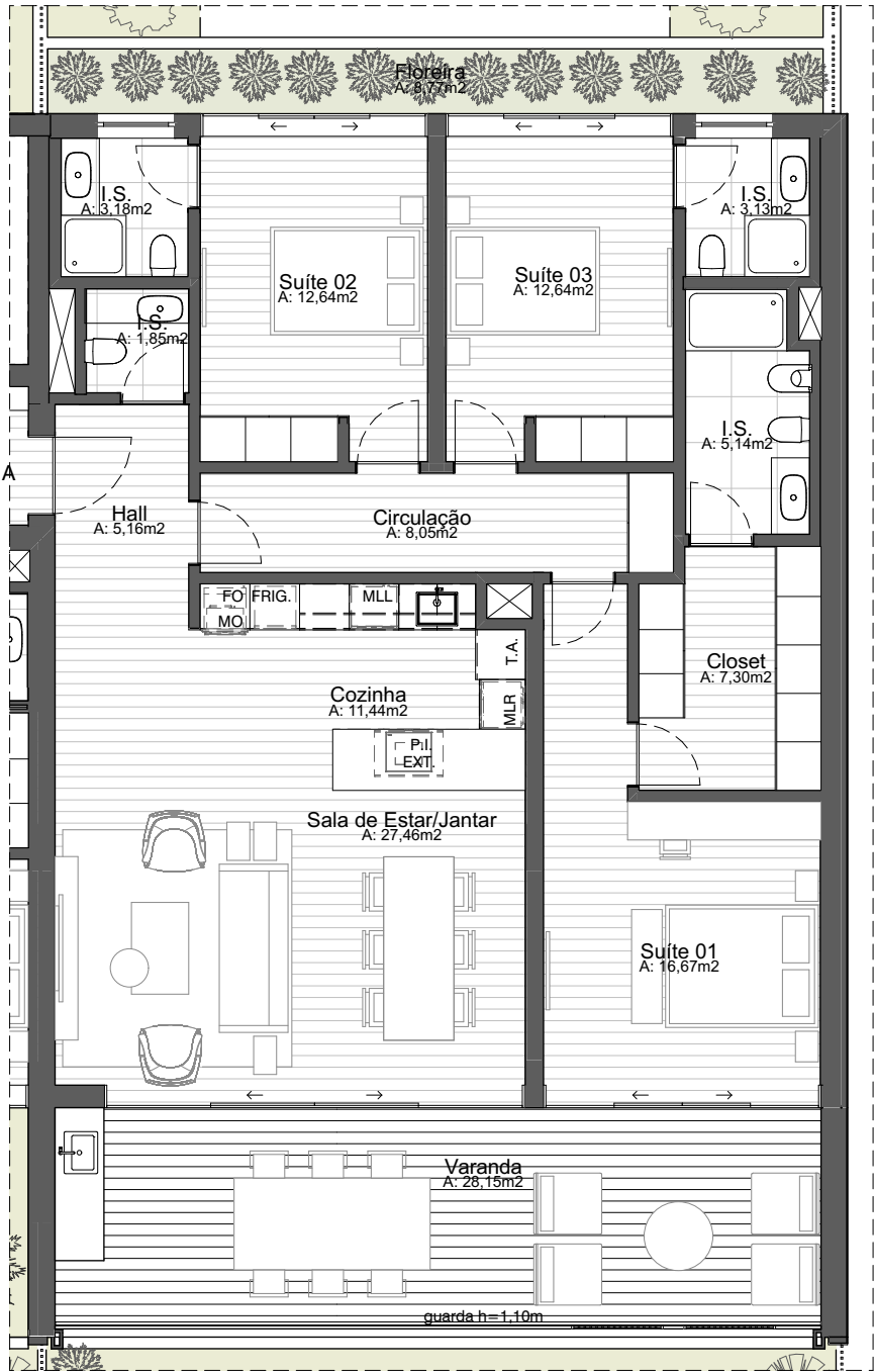
PLANTA - APARTAMENTO 0A 1:100
