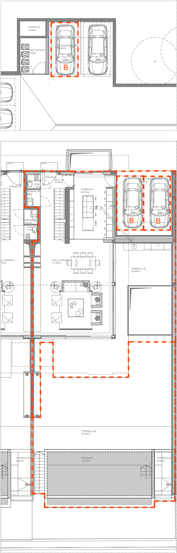
PLANTA DO PISO 0
