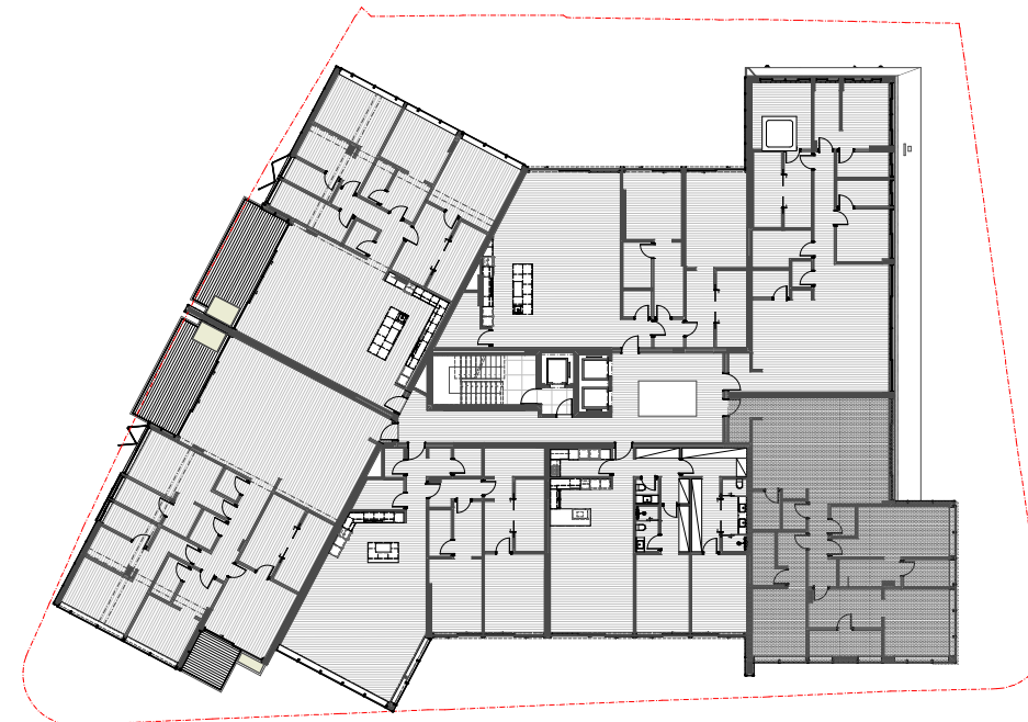
PLANTA ESQUEMÁTICA 1:500
