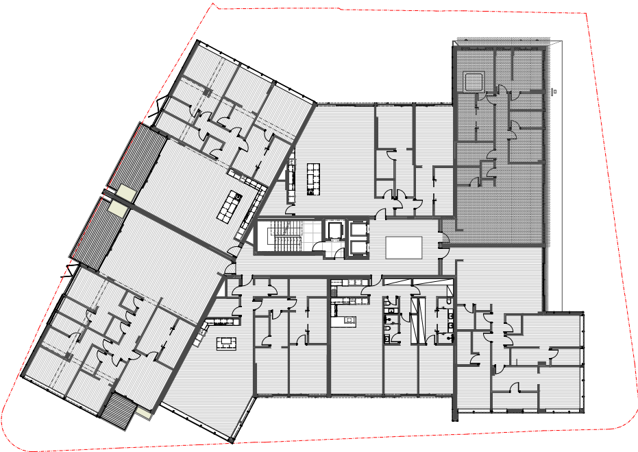
PLANTA ESQUEMÁTICA 1:500
