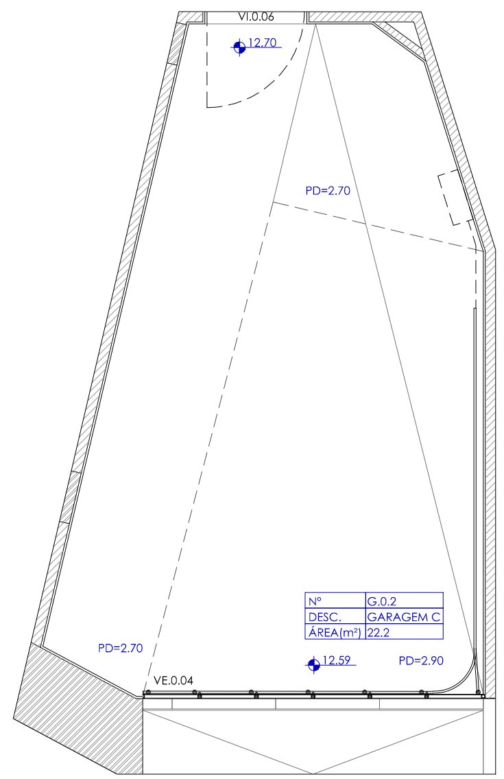
PLANTA GARAGEM FRACÇÃO C A.B.C. 27,65 m²
