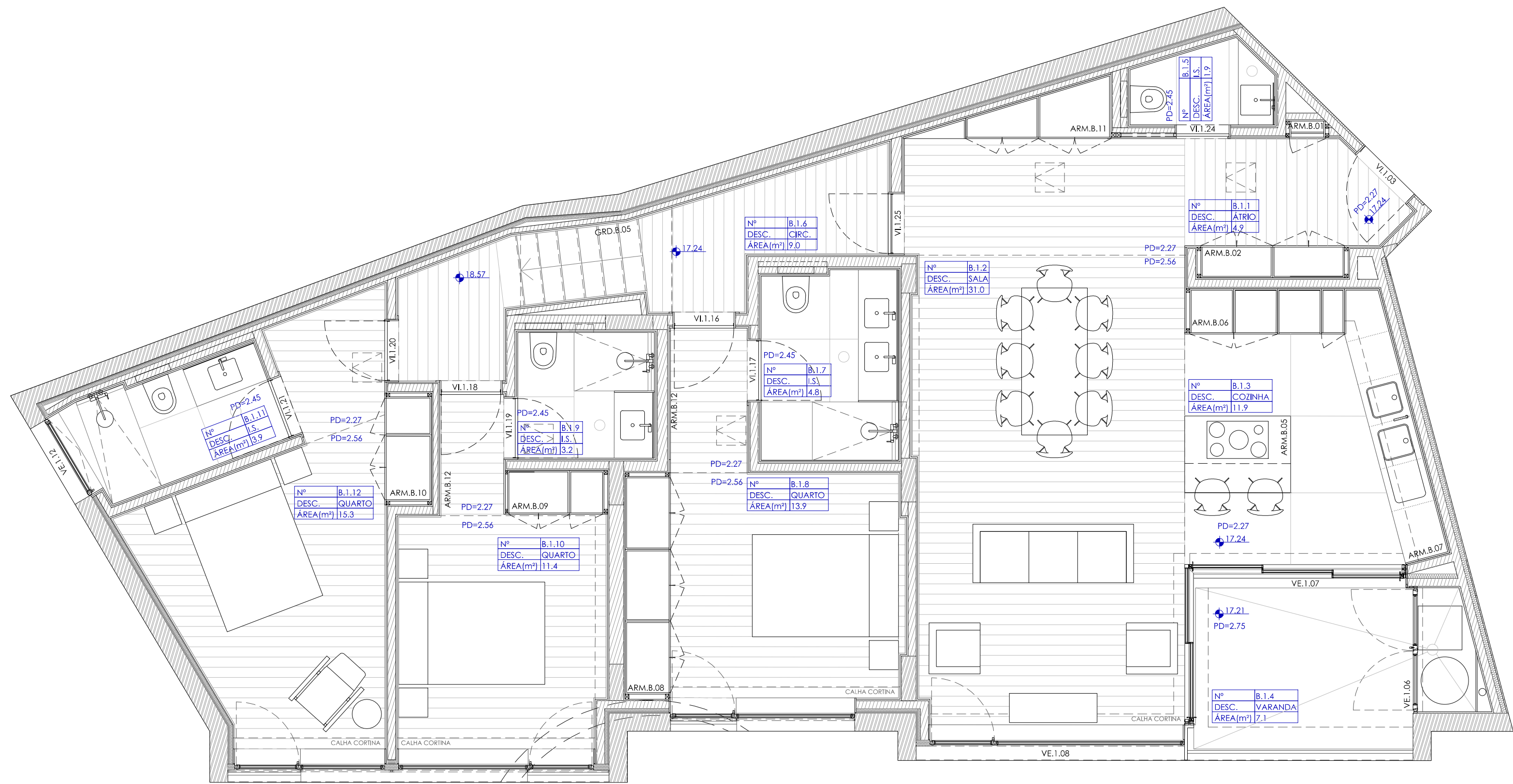
PLANTA FRACÇÃO B TIPOLOGIA T3 A.B.C. 148,64 m²
