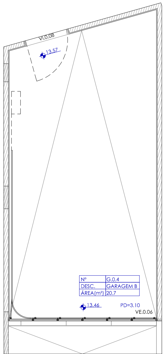
PLANTA GARAGEM FRACÇÃO B A.B.C. 25,41 m²
