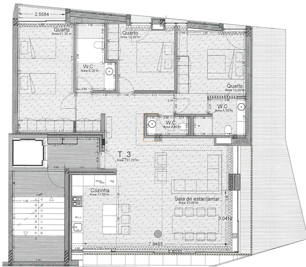
PLANTA DO 5.º PISO
