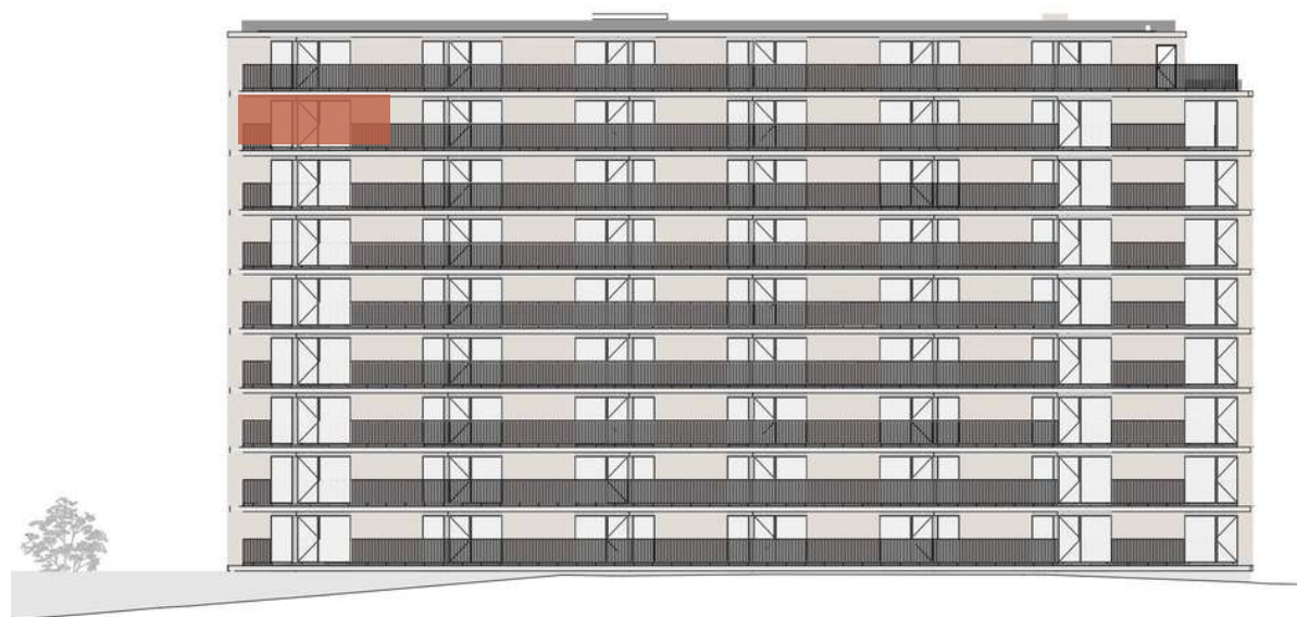
ALÇADO PRINCIPAL
