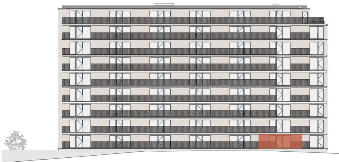
ALÇADO PRINCIPAL
