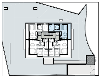
PLANTA DE LOCALIZAÇÃO piso 6
