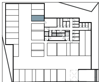
PLANTA DA GARAGEM piso -1
